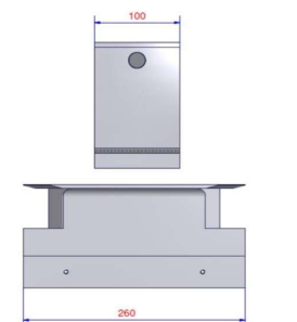
Fensterbankeinsatz Standard
