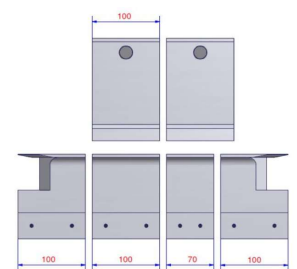
Fensterbankeinsatz Variabel
