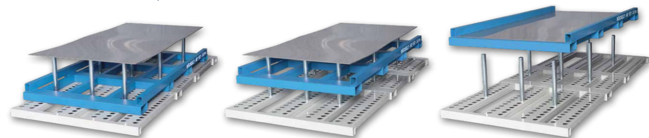
Funktionsweise des Entpalettierers
